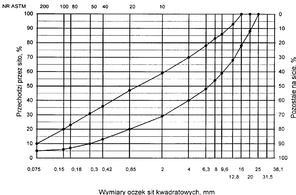
Rys. 1. Krzywe graniczne uziarnienia mieszanki mineralnej BA od 0 do 20 mm do warstwy ścierniczej nawierzchni drogi o obciążeniu ruchem dla KR1 lub KR2
