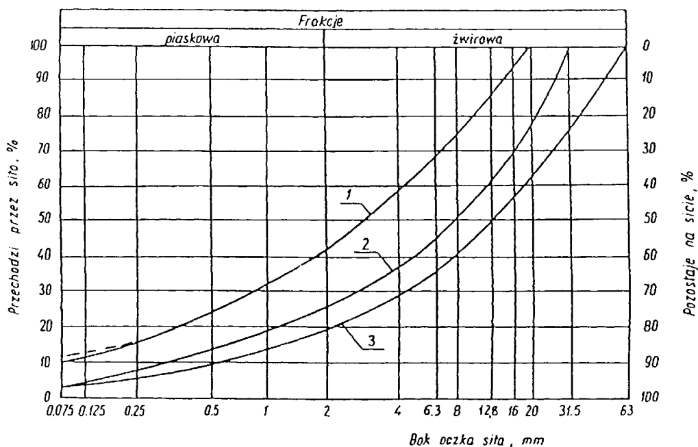
Rysunek 1. Pole dobrego uziarnienia kruszyw
